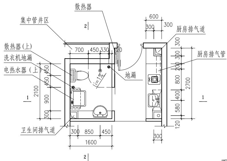
平面图
