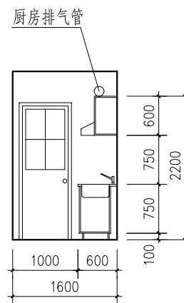
2-2剖面图
