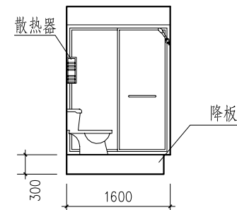
3-3剖面图
